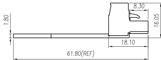
08~24P尺寸图
