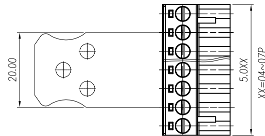
04~07P尺寸图
