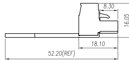
04~07P尺寸图
